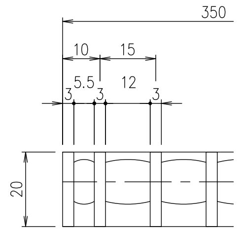
メインバーピッチ詳細図 S=1/1
