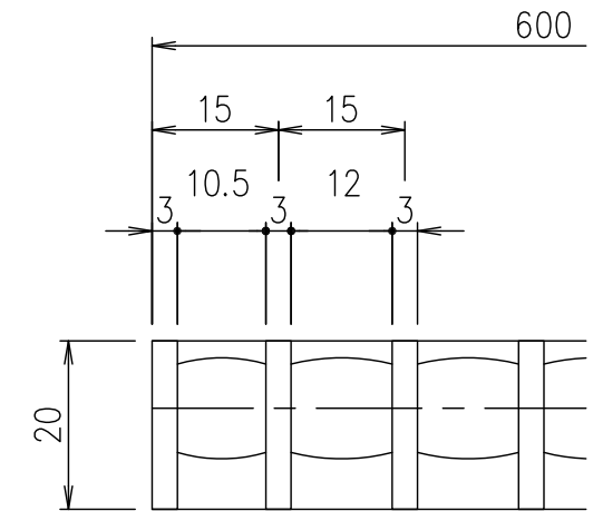
メンバーピッチ詳細図 S=1/1
