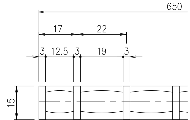
メインバーピッチ詳細図 S=1/1
