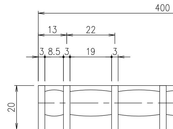
メインバーピッチ詳細図 S=1/1
