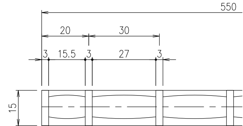
メインバーピッチ詳細図 S=1/1
