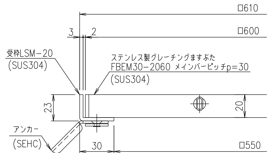
受棒断面詳細図 S=1/2
