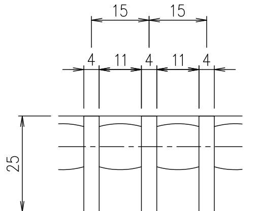
メンバーピッチ詳細図 S=1/1
