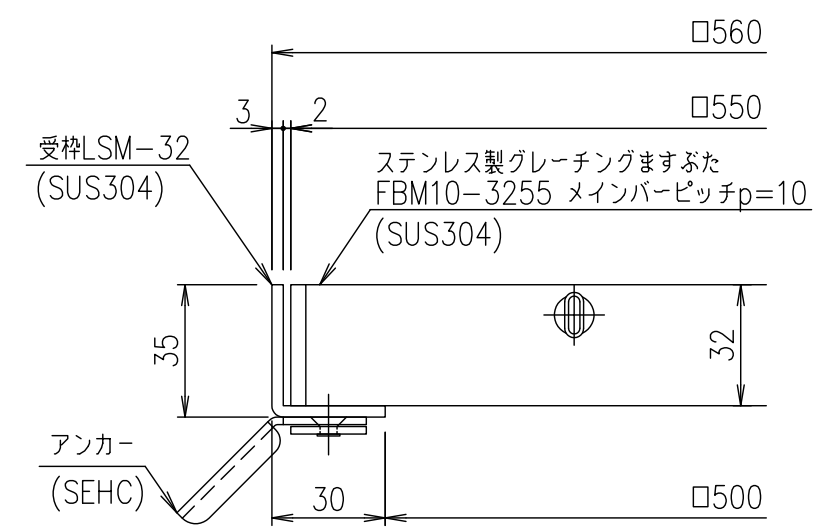
受枠断面詳細図 S=1/2
