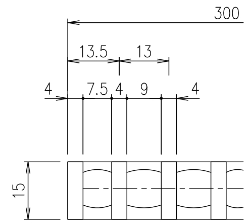
メインバーピッチ詳細図 S=1/1
