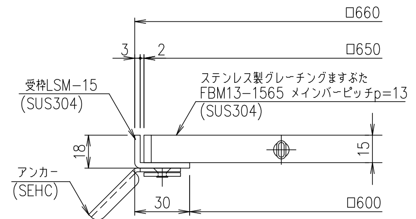
受枠断面詳細図 S=1/2
