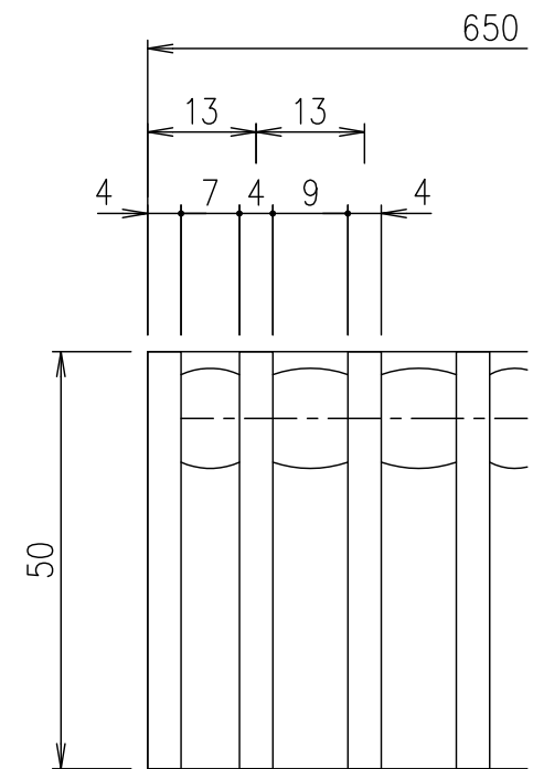
メンバーピッチ詳細図 S=1/1
