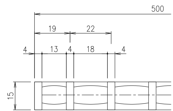
メインバーピッチ詳細図 S=1/1
