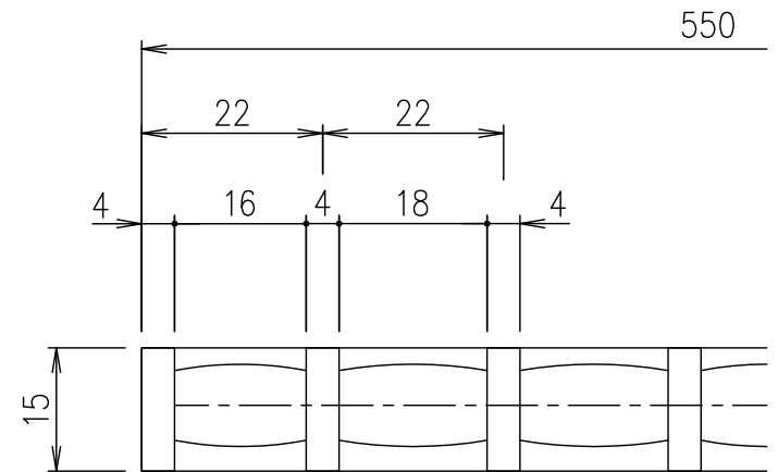
メインバーピッチ詳細図 S=1/1
