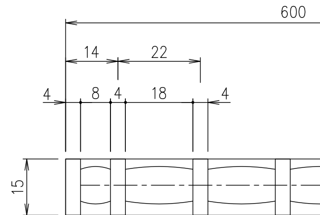
メインバーピッチ詳細図 S=1/1
