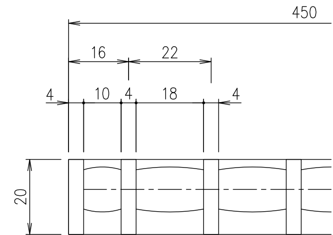
メンバーピッチ詳細図 S=1/1
