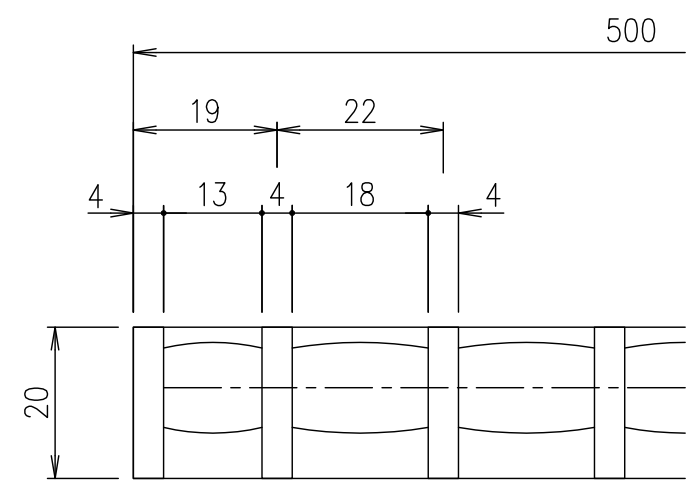
メインバーピッチ詳細図 S=1/1
