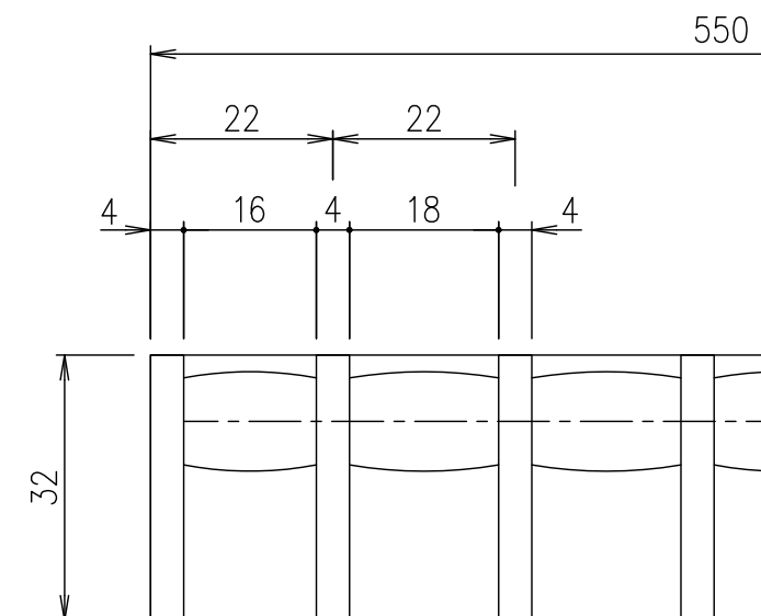
メインバーピッチ詳細図 S=1/1
