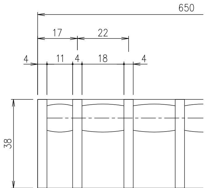
メンバーピッチ詳細図 S=1/1
