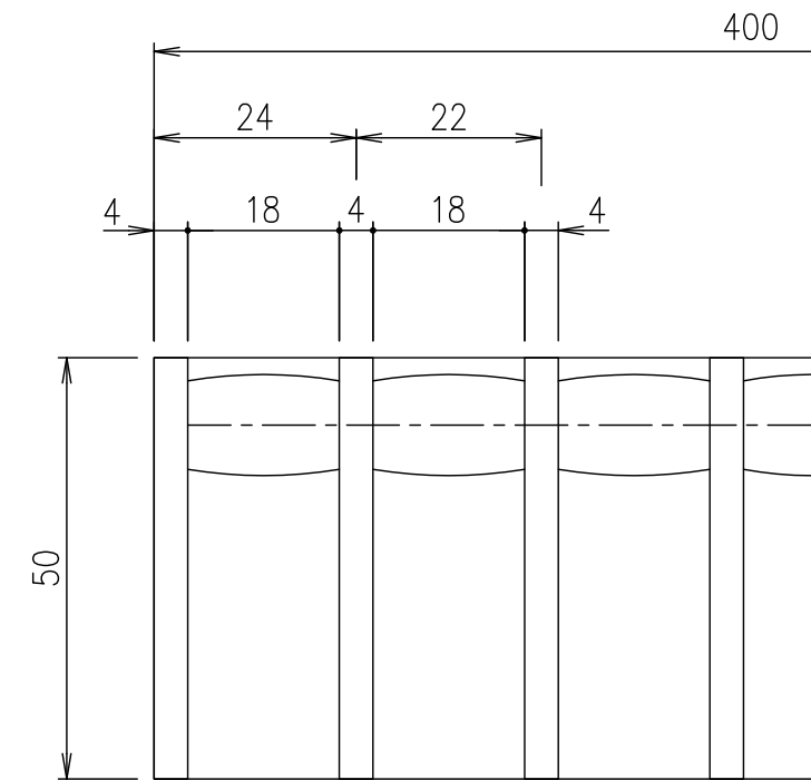
□410 □400 3 2 受枠LSM-50 (SUS304) ステンレス製グレーチングますぶた FBM22-5040 メインバーピッチ p=22 (SUS304) 53 50 アンカー (SEHC) 30 □350
