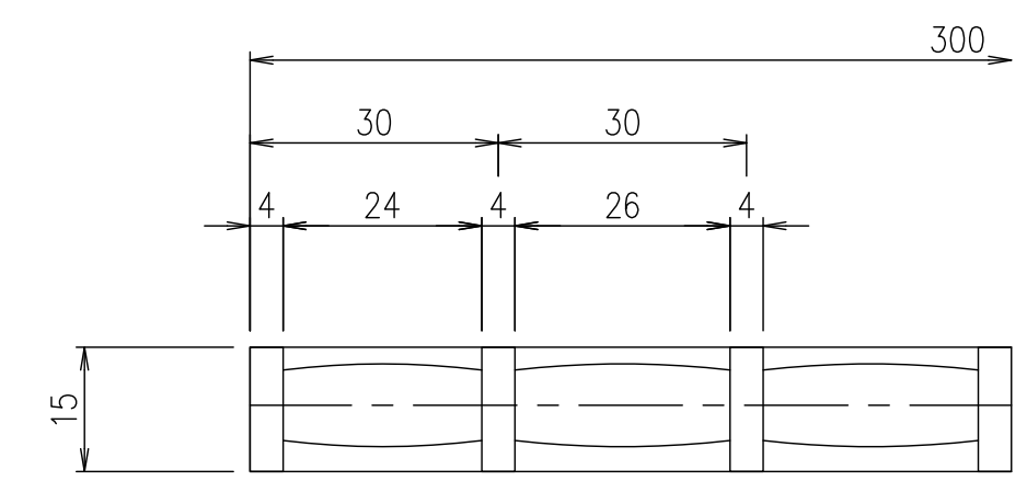
メインバーピッチ詳細図 S=1/1
