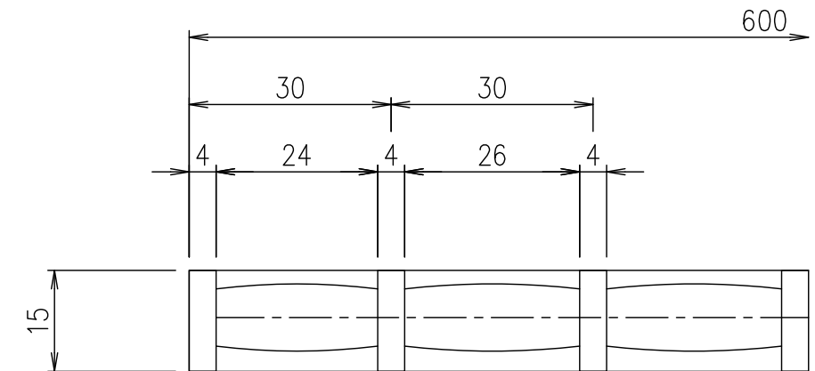
メインバーピッチ詳細図 S=1/1
