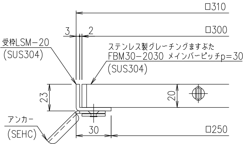
受枠断面詳細図 S=1/2
