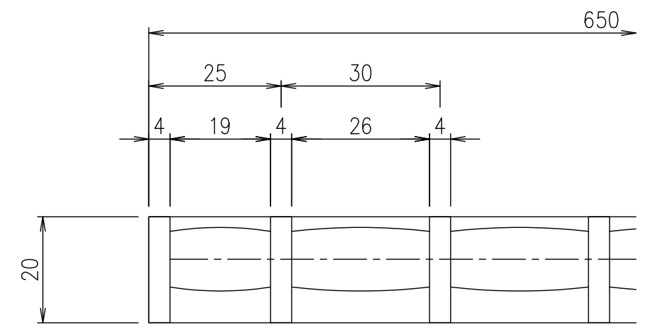
メインバーピッチ詳細図 S=1/1
