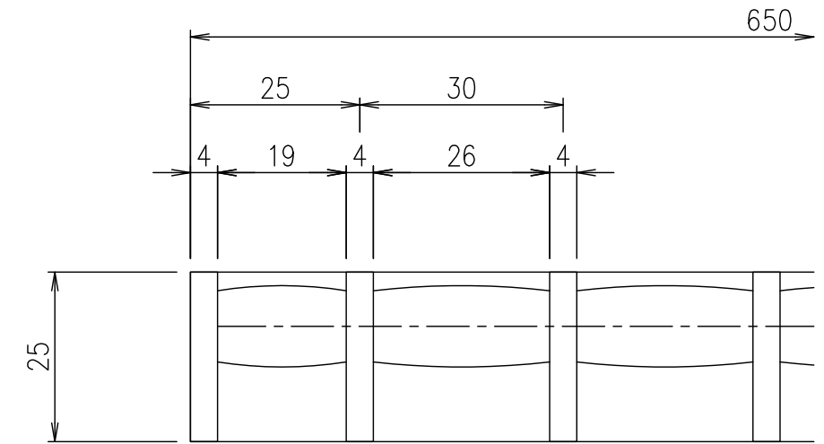
メンバーピッチ詳細図 S=1/1
