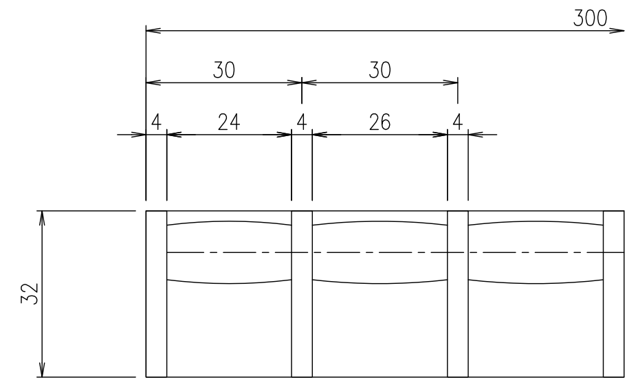
メンバーピッチ詳細図 S=1/1
