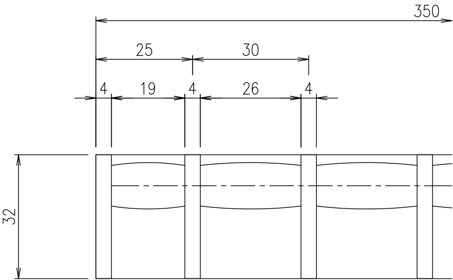
メインバーピッチ詳細図 S=1/1
