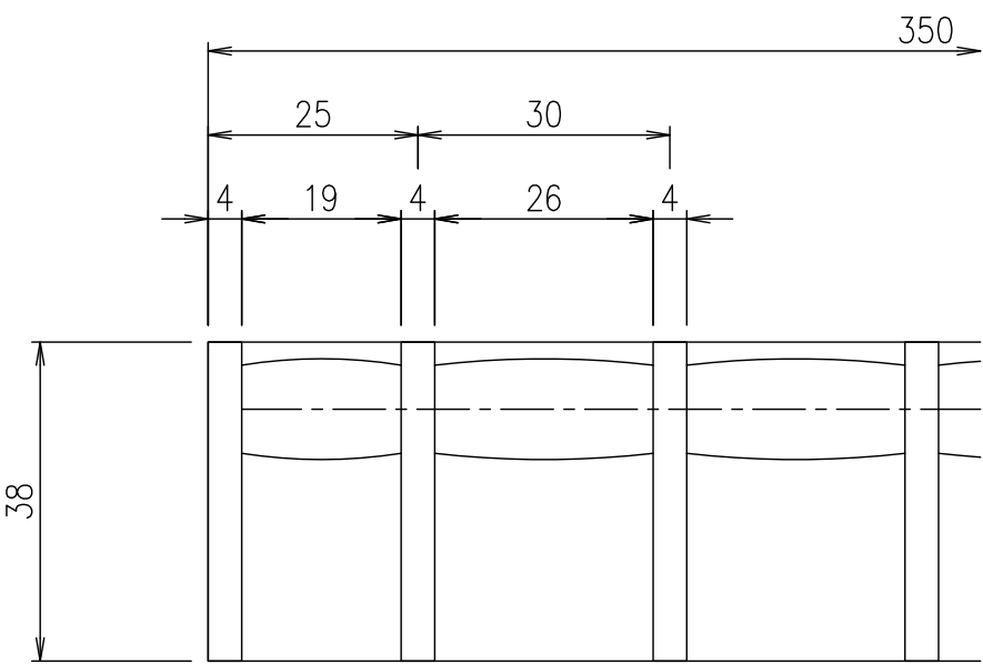
メインバーピッチ詳細図 S=1/1
