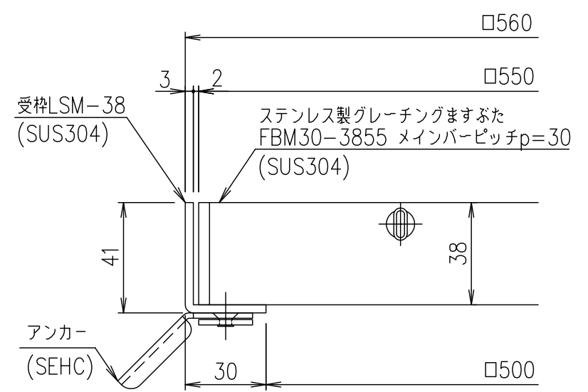
受枠断面詳細図 S=1/2
