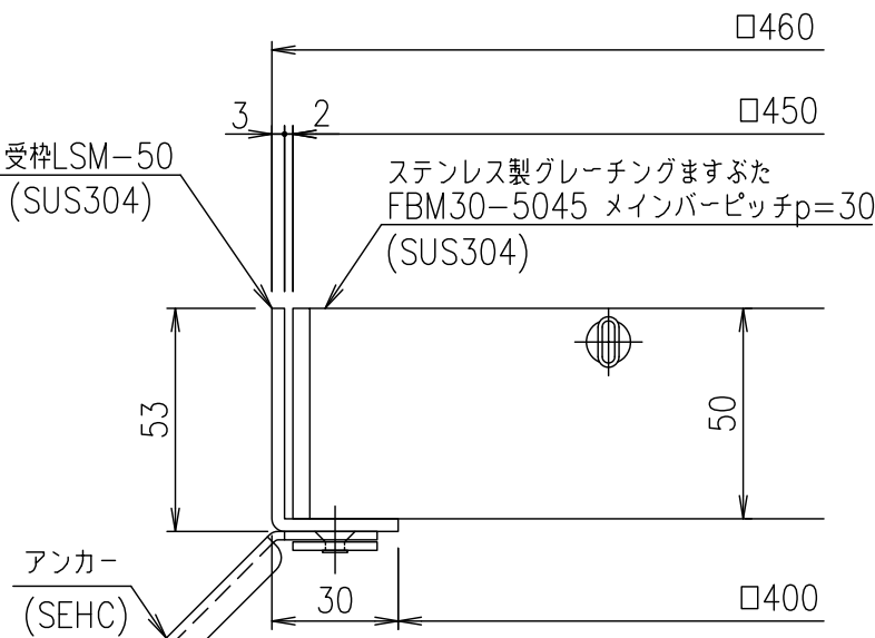
受枠断面詳細図 S=1/2
