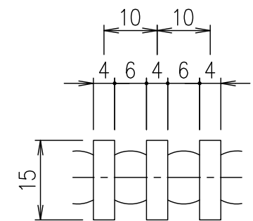
メンバーピッチ詳細図 S=1/1
