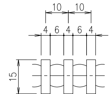
メンバーピッチ詳細図 S=1/1
