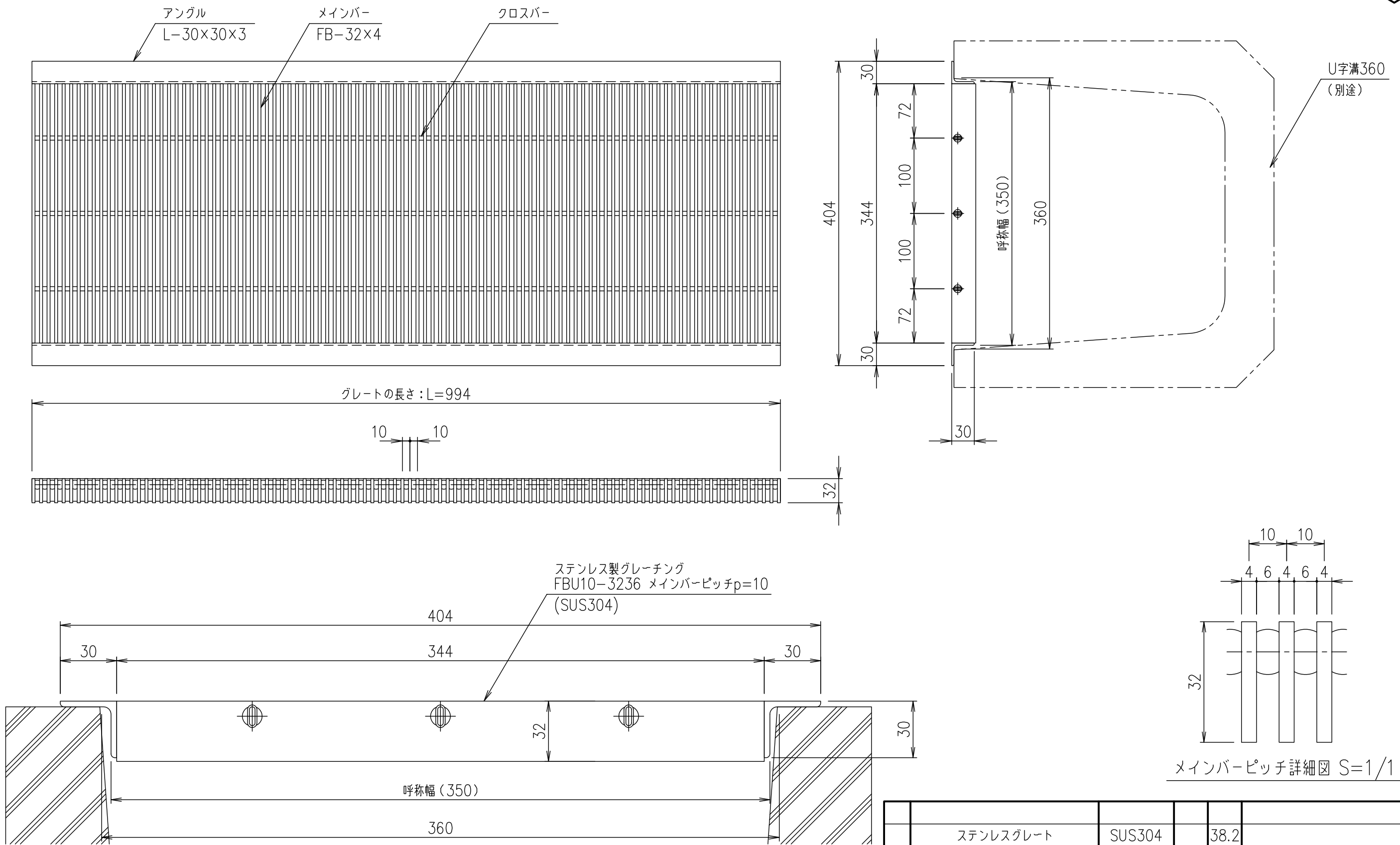
断面詳細図 S=1/2
