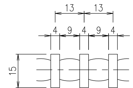
メンバーピッチ詳細図 S=1/1
