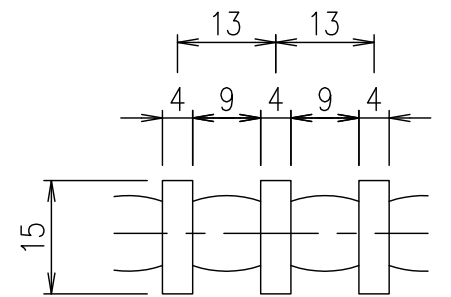
メインバーピッチ詳細図 S=1/1
