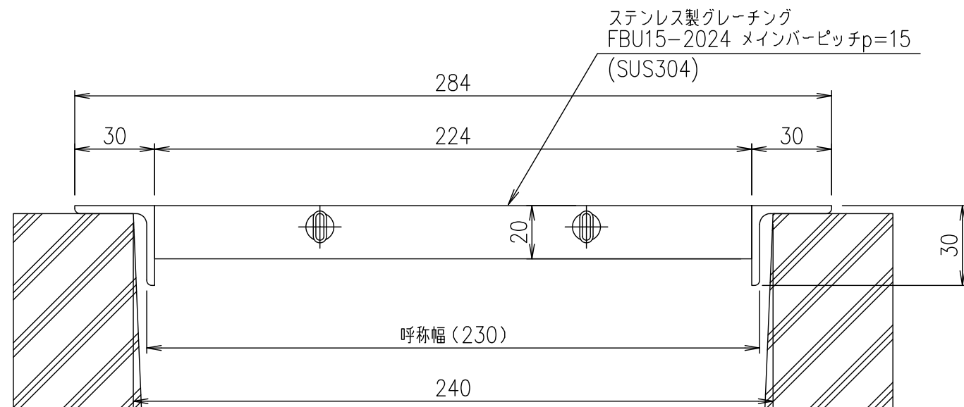
断面詳細図 S=1/2
