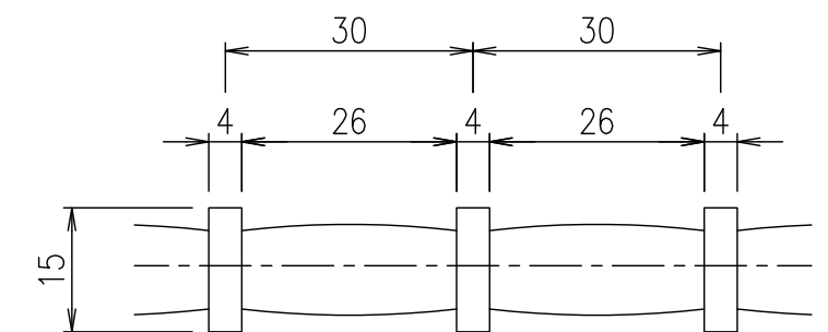
メインバーピッチ詳細図 S=1/1
