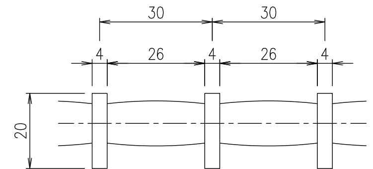
メンバーピッチ詳細図 S=1/1
