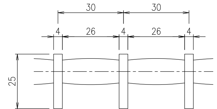
メンバーピッチ詳細図 S=1/1
