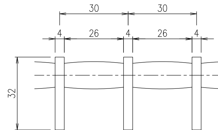
メインバーピッチ詳細図 S=1/1
