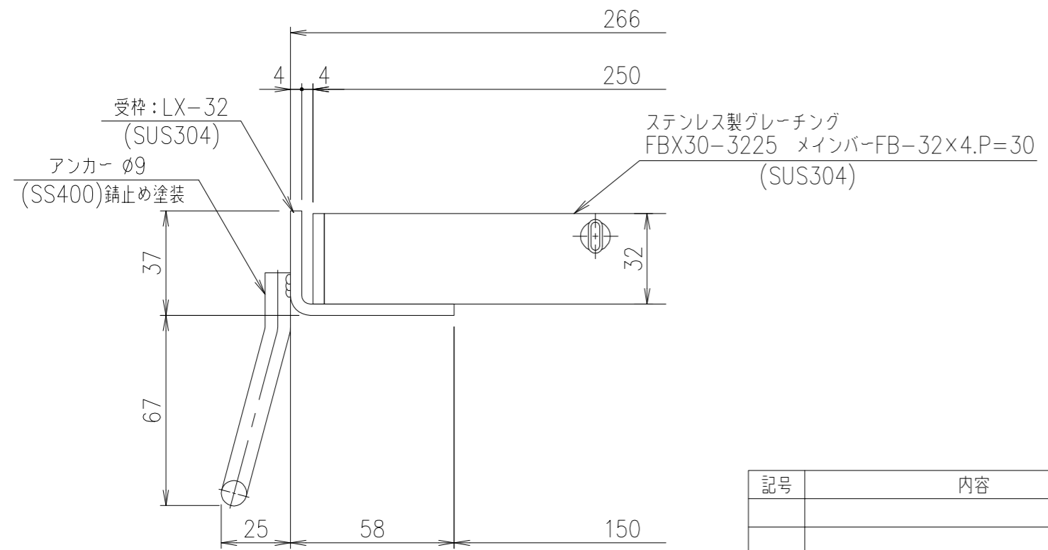
受枠断面詳細図 S=1/2
