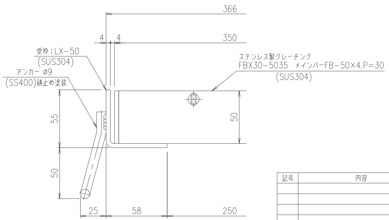
受枠断面詳細図 S=1/2
