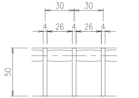
メインバーピッチ詳細図 S=1/2
