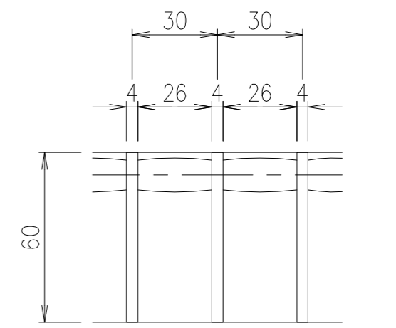
メインバーピッチ詳細図 S=1/2
