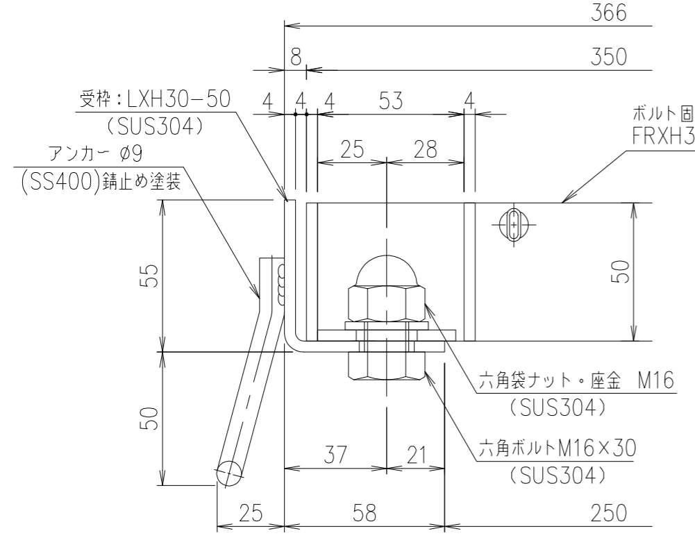
受枠断面詳細図 S=1/2
