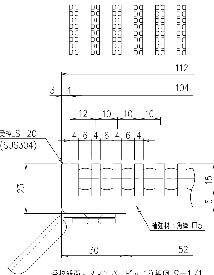
受枠断面・メインバーピッチ詳細図 S=1/1
