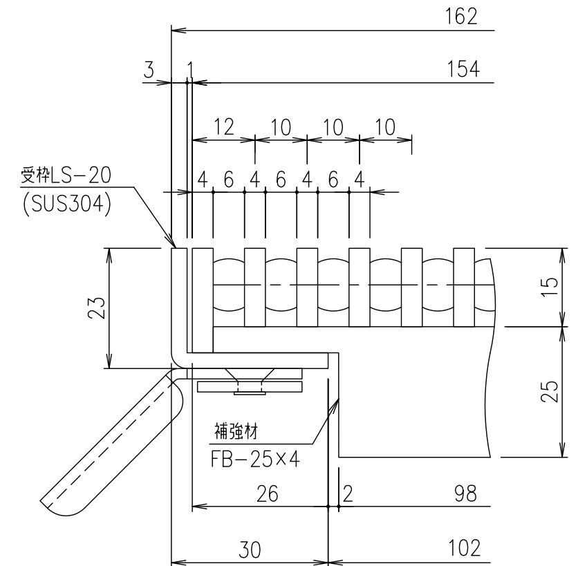
受枠断面・メンバーピッチ詳細図 S=1/1
