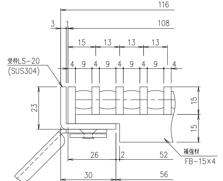
受枠断面・メインバーピッチ詳細図 S=1/1
