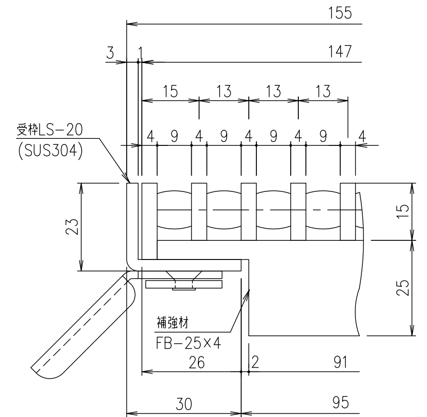
受枠断面・メインバーピッチ詳細図 S=1/1
