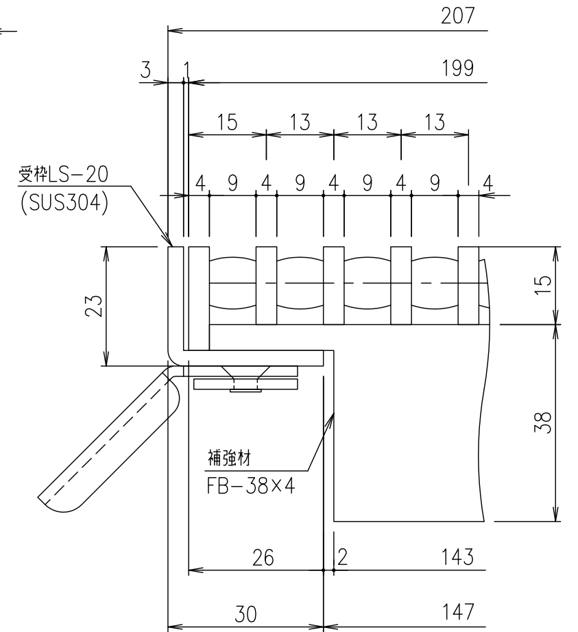
受枠断面・メインバーピッチ詳細図 S=1/1
