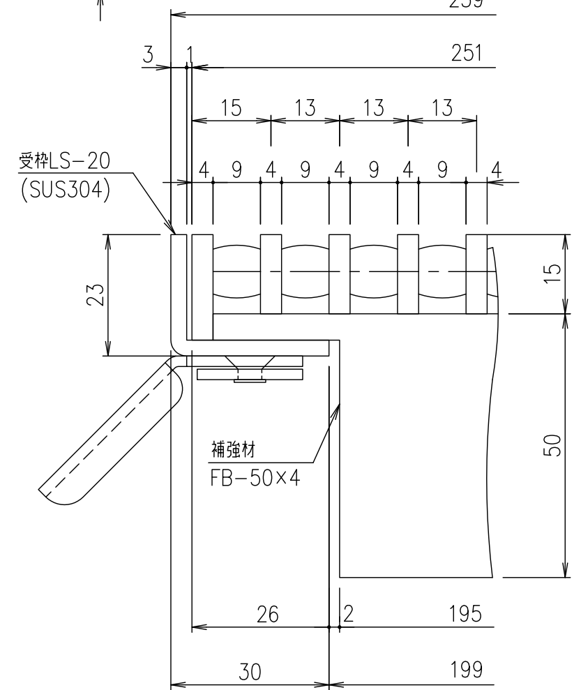
受枠断面・メインバーピッチ詳細図 S=1/1
