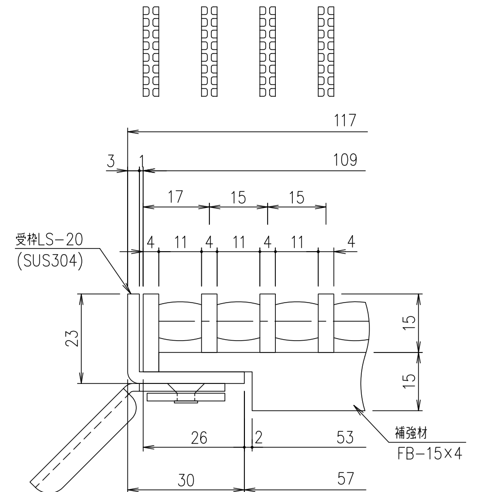
受枠断面。メインバーピッチ詳細図 S=1/1
